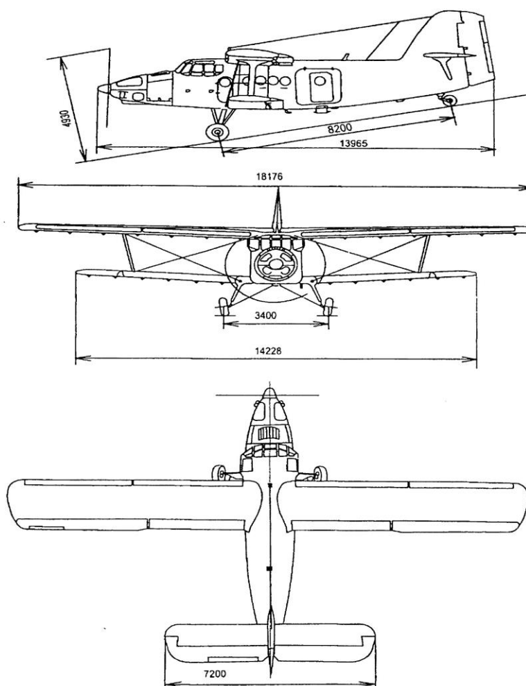
Рис. 61 Самолет Ан-3Т
