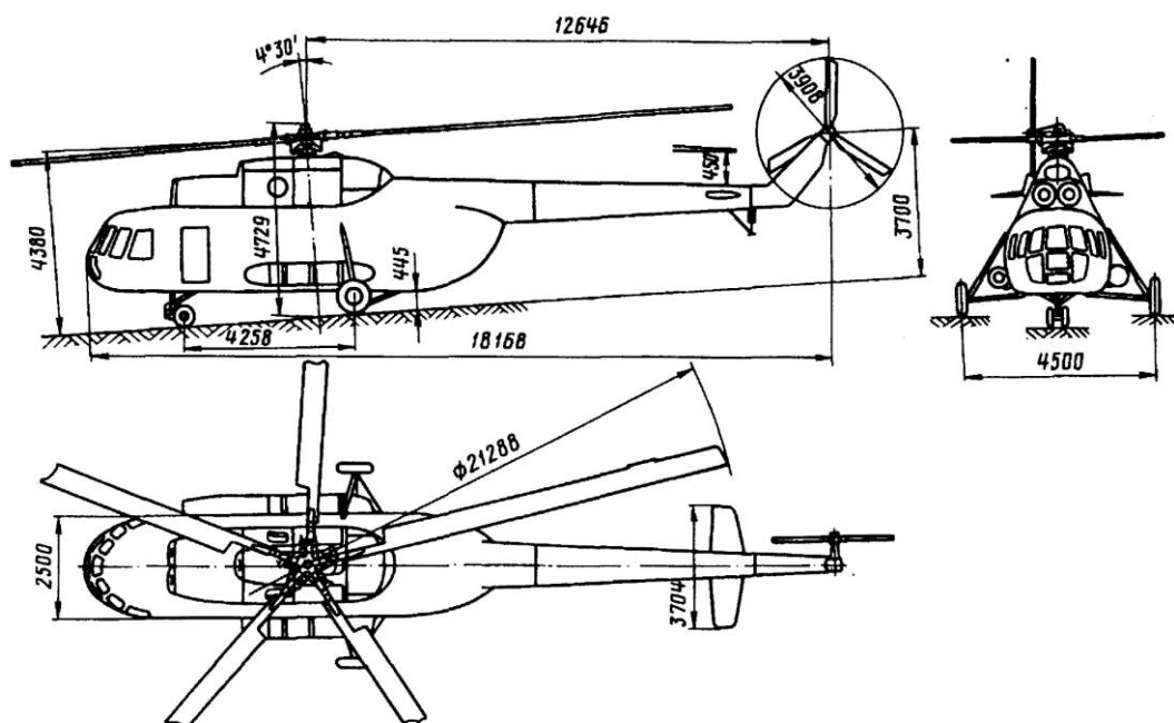
Рис. 59 Вертолет Ми-8Т
