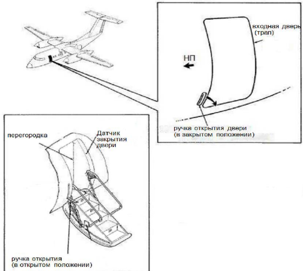
Рис.32 Открытие/закрытие переднего трапа-двери снаружи
