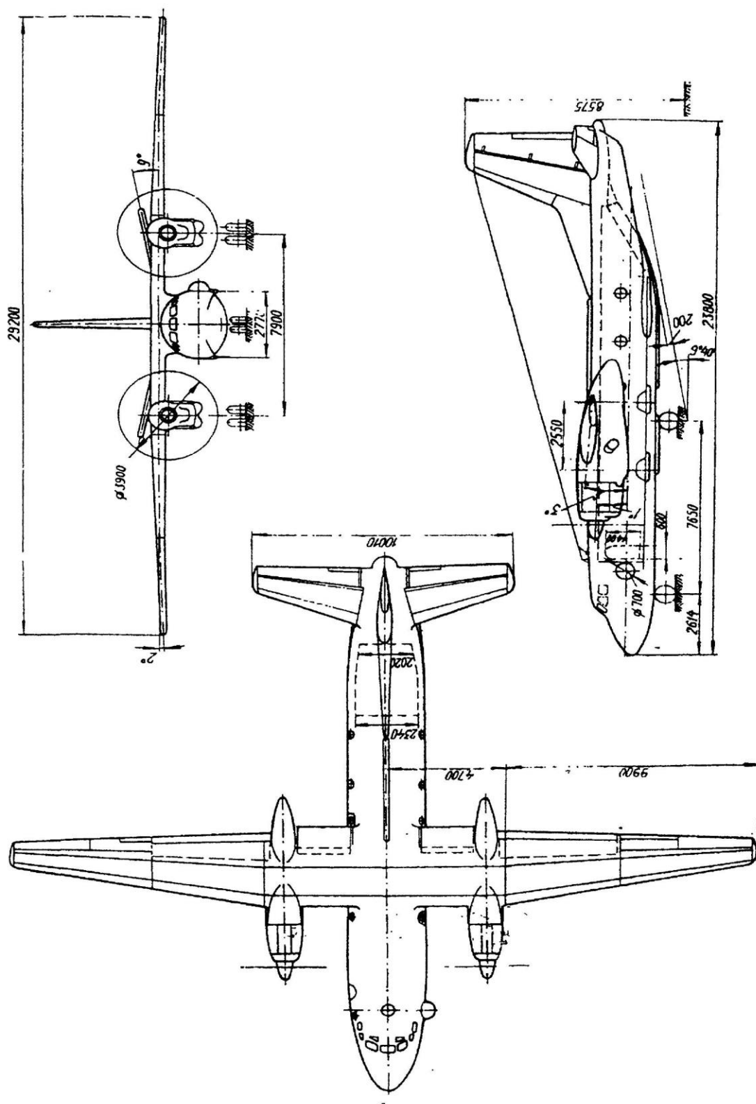
Рис. 56 Самолет Ан-26
