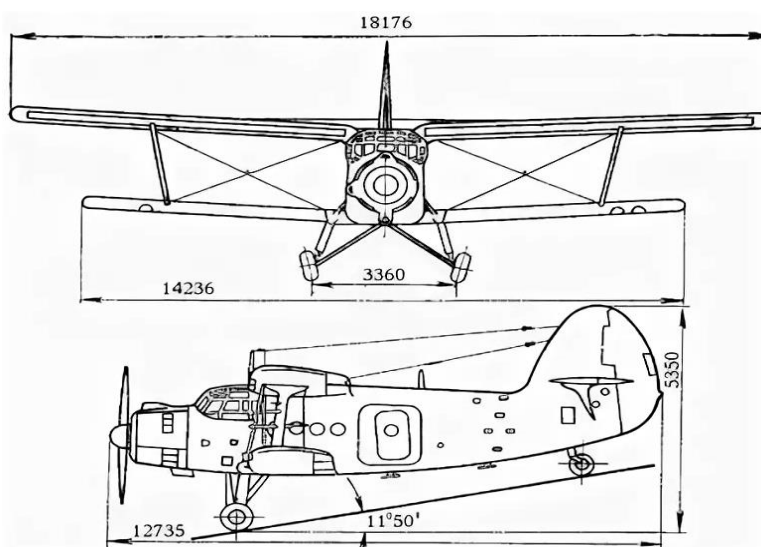
Рис. 60 Самолет Ан-2
