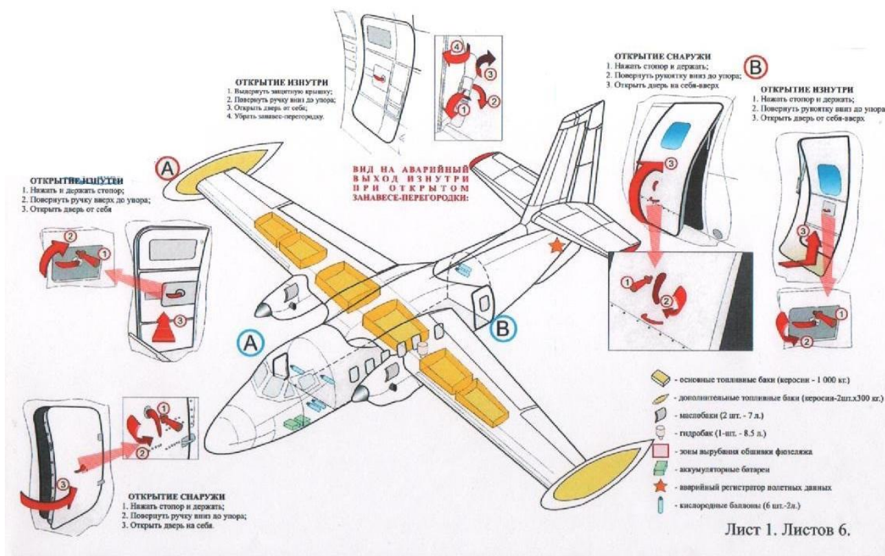
Рис. 19 Порядок открывания дверей и люков на ВС Л-410УВП-Э
