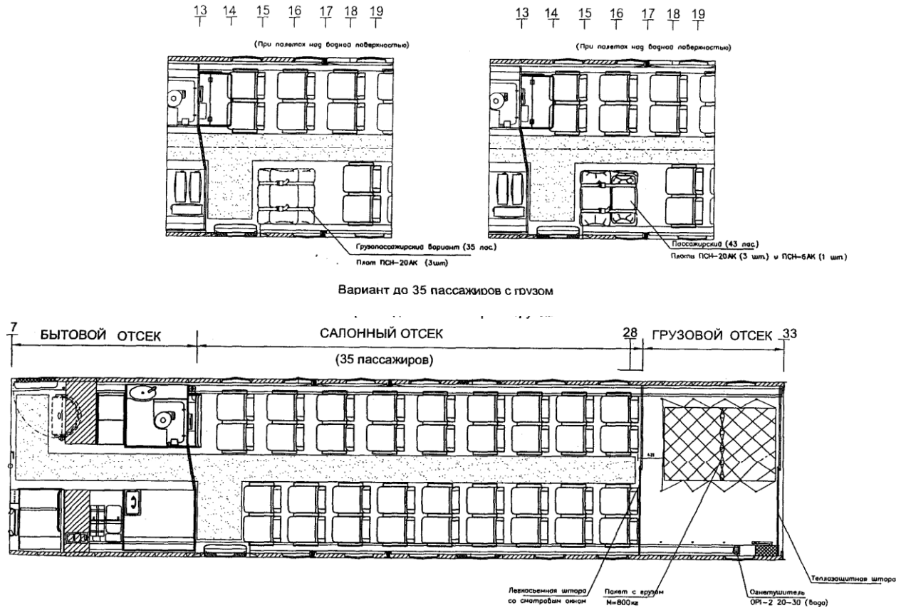
Рис. 5 Вариант до 35 пассажиров с грузом
