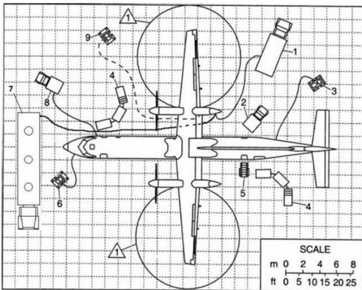
△1 - во время заправки держать зоны свободными Рис.106 Схема подъезда (отъезда) и маневрирования спецмашин при обслуживании воздушного судна Bombardier DHC-8-300.
