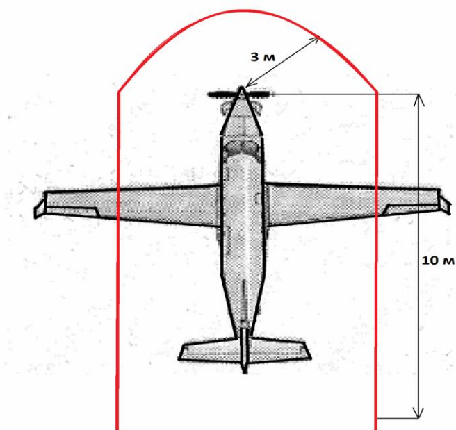
Рис. 43 Схема опасных зон ВС Pilatus PC -6/B2-H4 при работе на максимальном взлетном режиме
