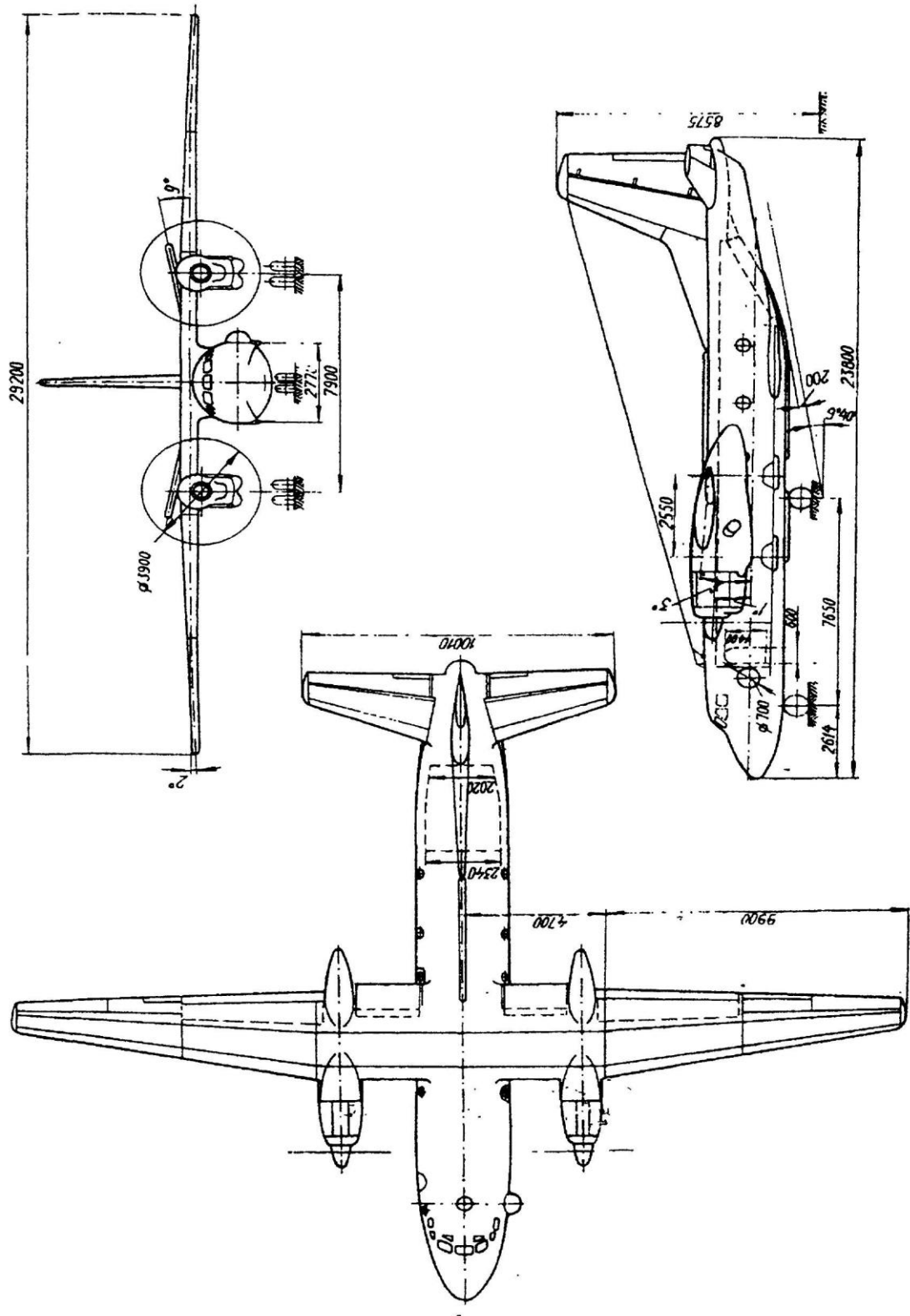
Рис. 56 Самолет Ан-26
