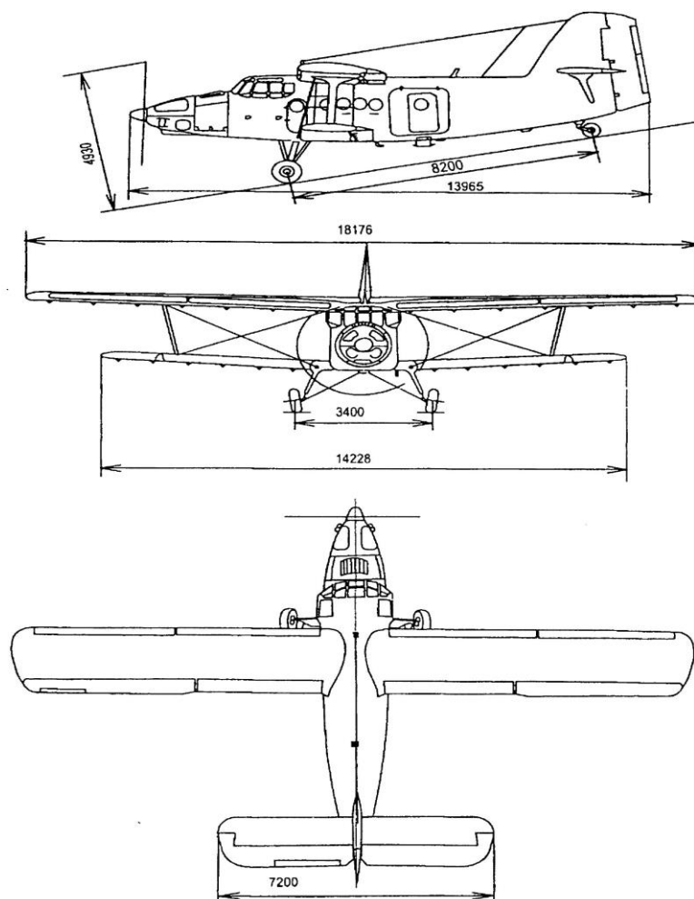
Рис. 61 Самолет Ан-3Т
