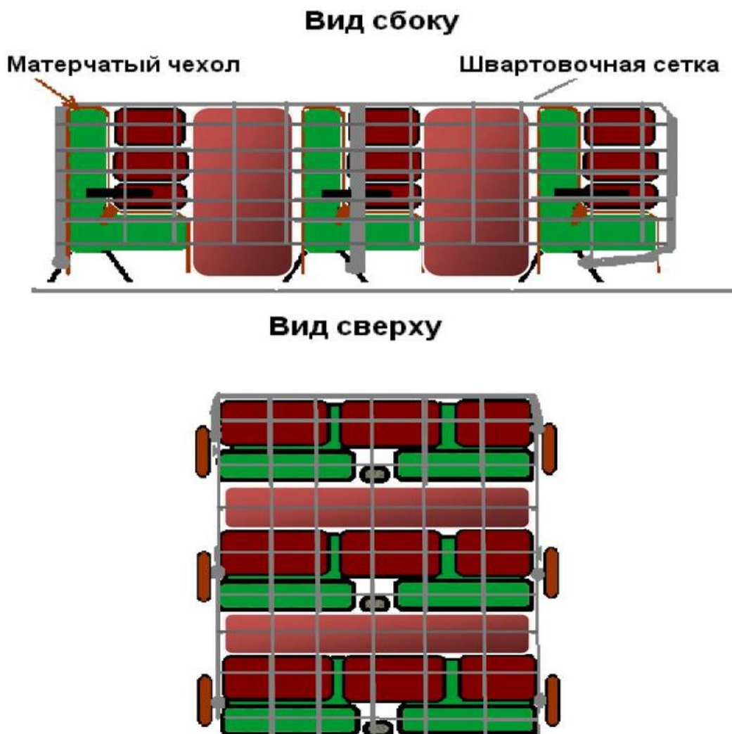
Схема размещения и крепления груза в пассажирском салоне ВС Ан-24/26.
