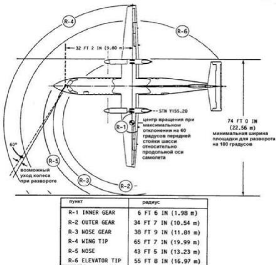
Рис. 92 Радиусы поворота.
