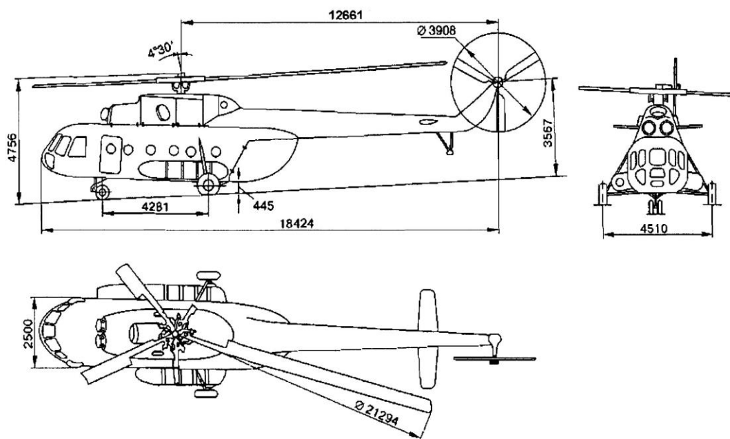
Рис. 58 Вертолет Ми-8МТВ-1
