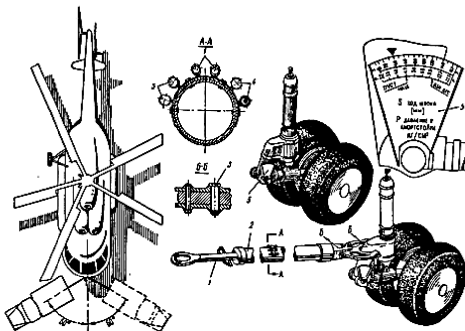
1—предохранительный болт BAT-9800-02; 2—штанга водила, 3—предохранительный болт BAT-9800-07, 4—предохранительный болт BAT-9800-15 буксировочного троса; 5—указатель хода штока и давления в амортизационной стойке
