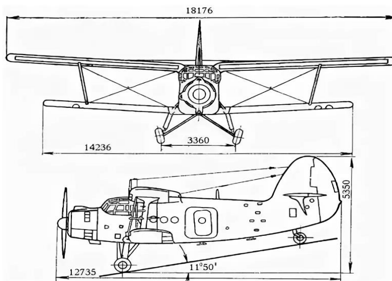
Рис. 60 Самолет Ан-2
