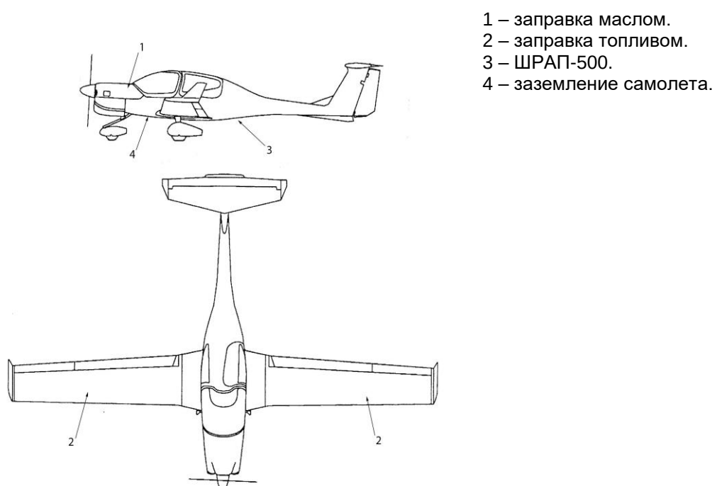
Рис. 51 Расположение точек наземного обслуживания самолета DA-40NG
