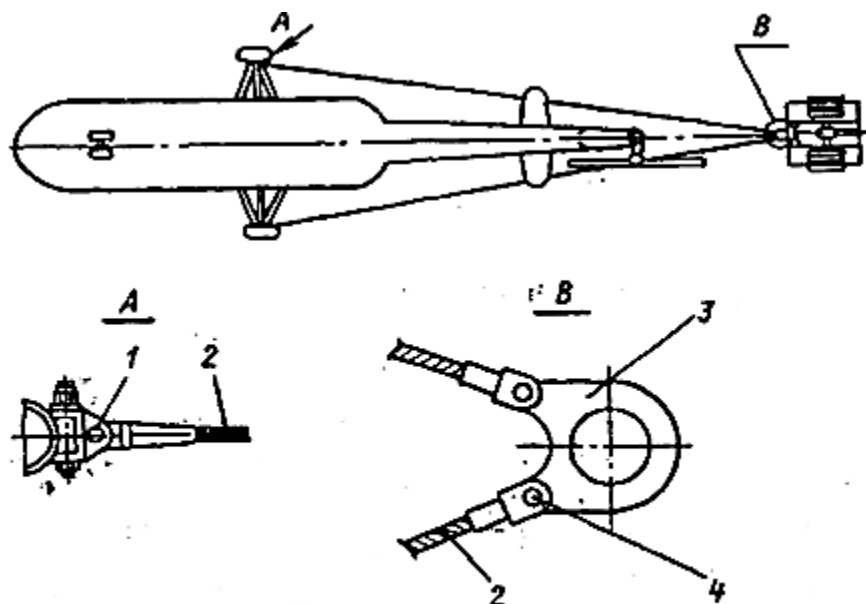
1. Кардан 2. Трос 3. Серьга 4. Предохранительный болт BAT-9800-15
