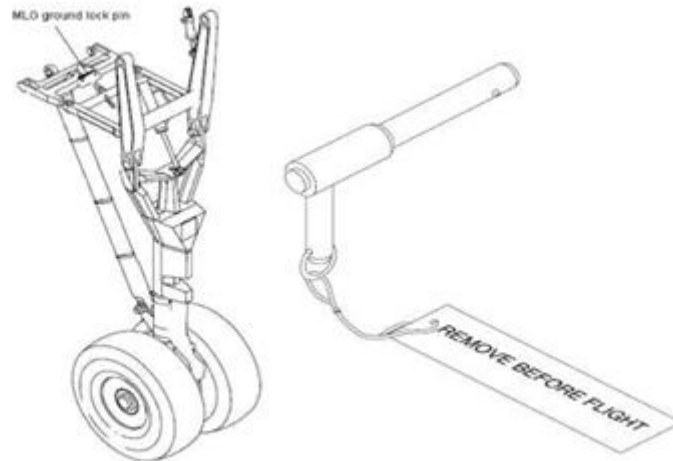
Рис. 94 Установка штырей (пинов) на замках выпущенного положения основных опор шасси.
