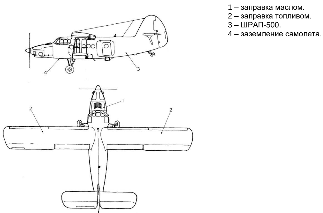
Рис. 50 Расположение точек наземного обслуживания самолета Ан-3Т
