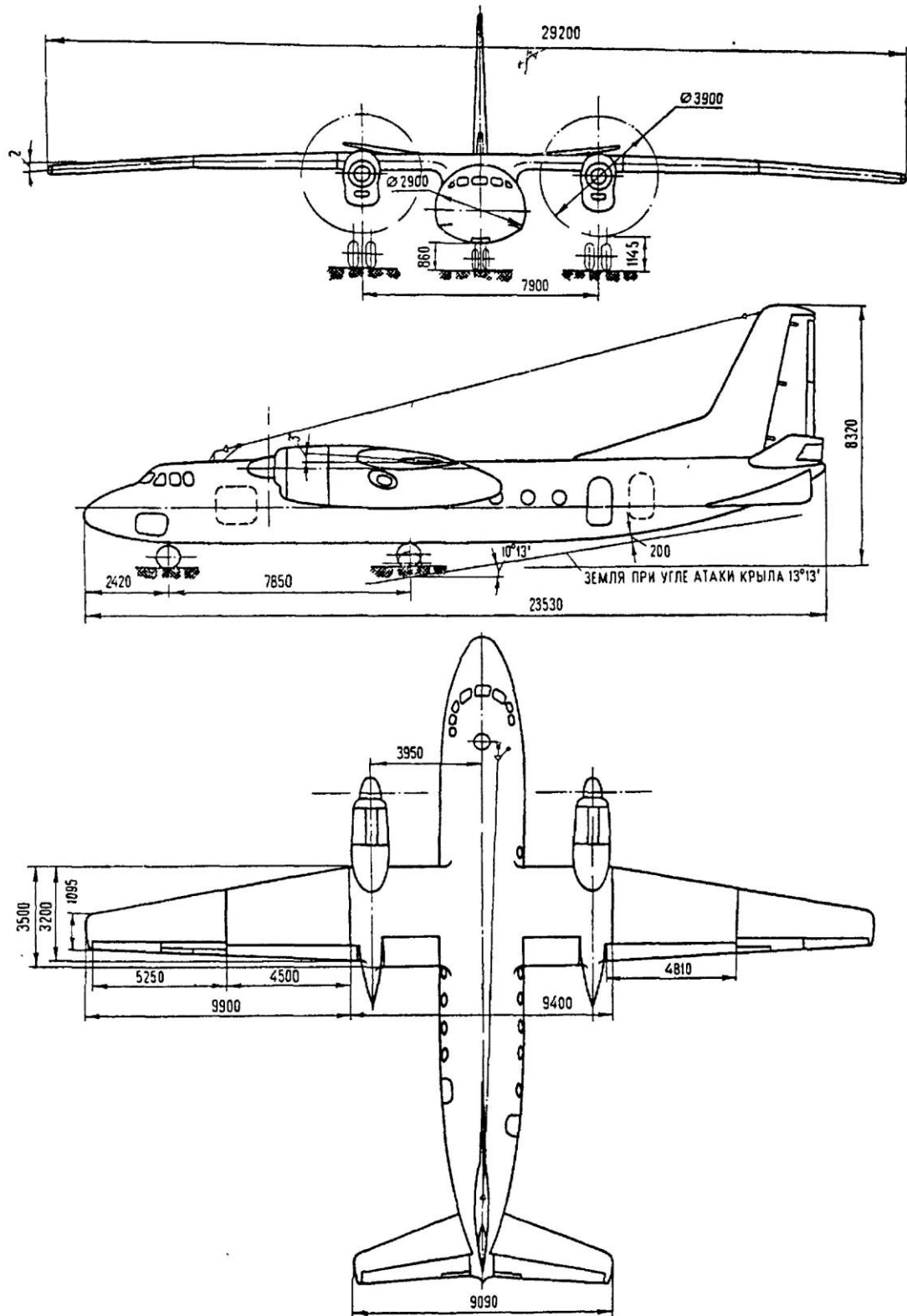
Рис. 55 Самолет Ан-24РВ
