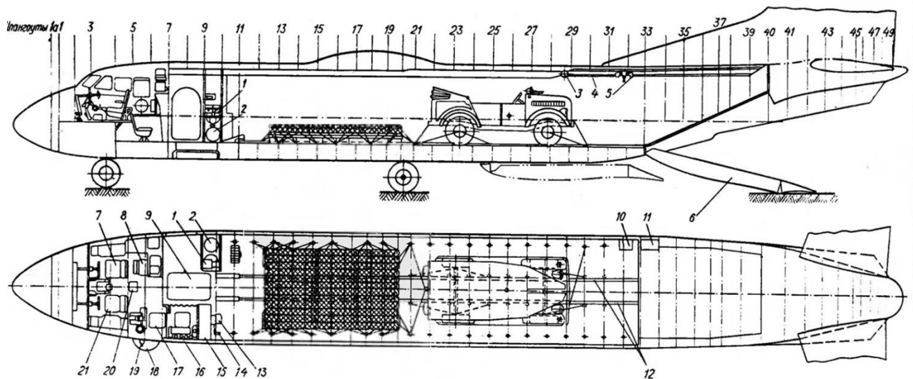
Рис. 2. Компоновочная схема кабин самолета:
