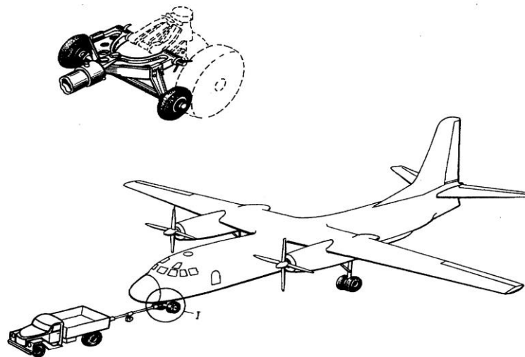
Рис. 82 Буксировка ВС
