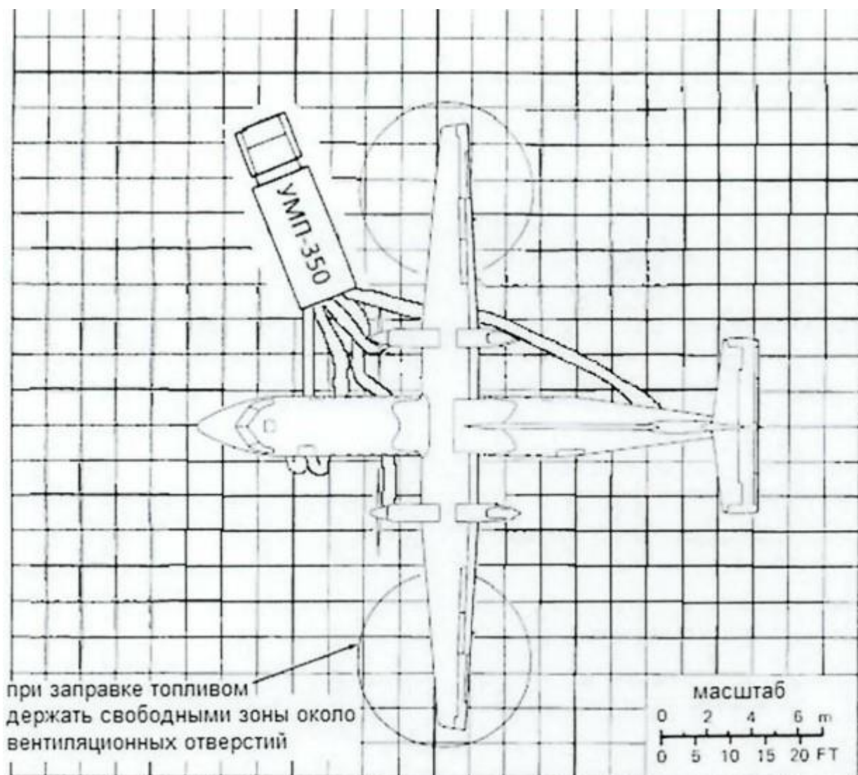
Рис. 81 Рекомендуемая схема расположения наземных подогревателей.
