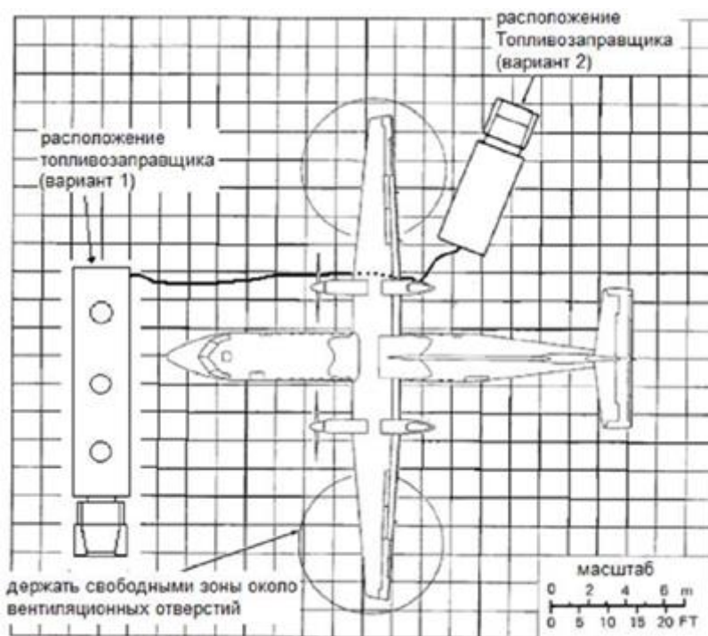
Рис. 74 Схема подъезда топливозаправочной машины.
