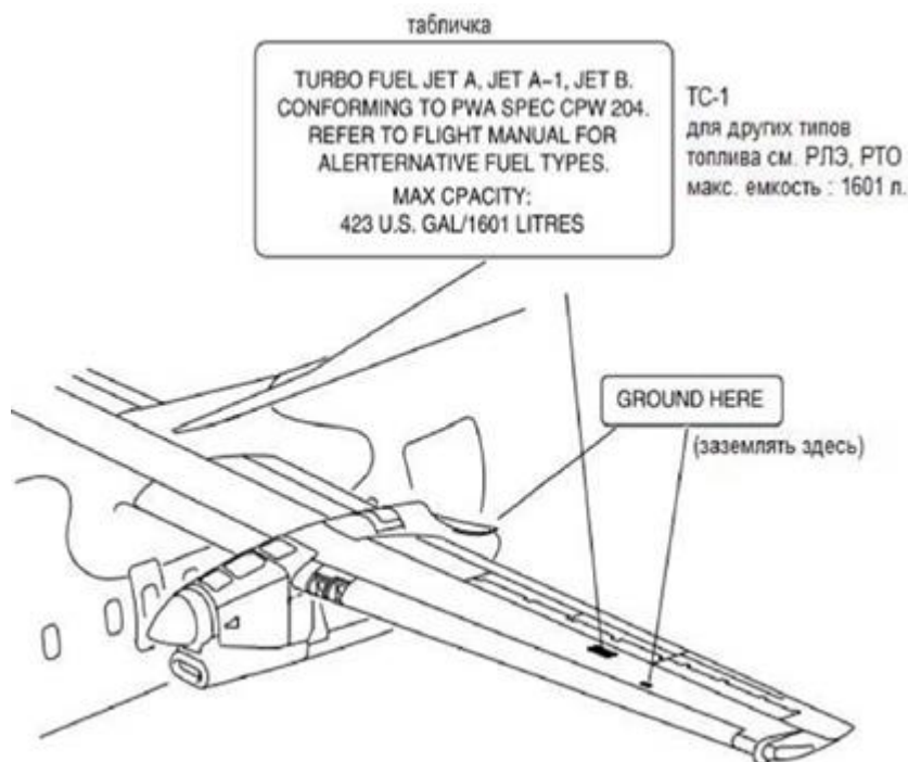
Рис.78 Таблички, надписи.
