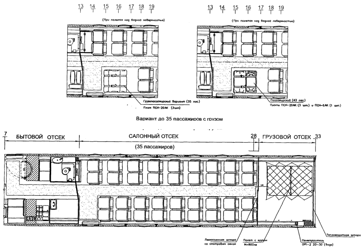
Рис. 5 Вариант до 35 пассажиров с грузом
