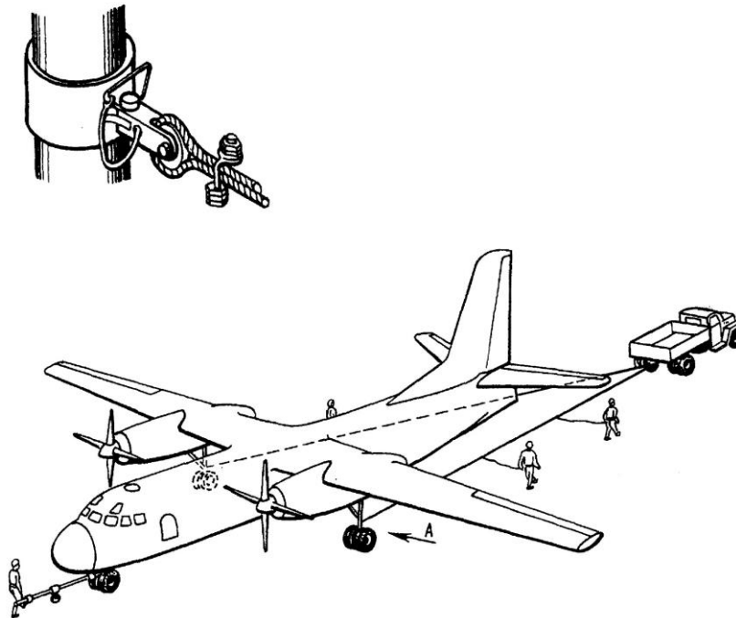
Рис.83 Буксировка ВС
