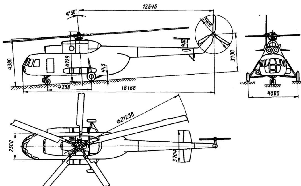
Рис. 59 Вертолет Ми-8Т
