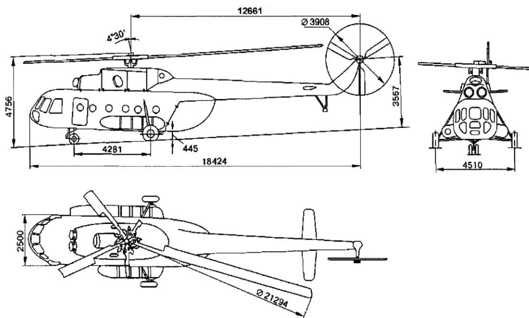
Рис. 58 Вертолет Ми-8МТВ-1
