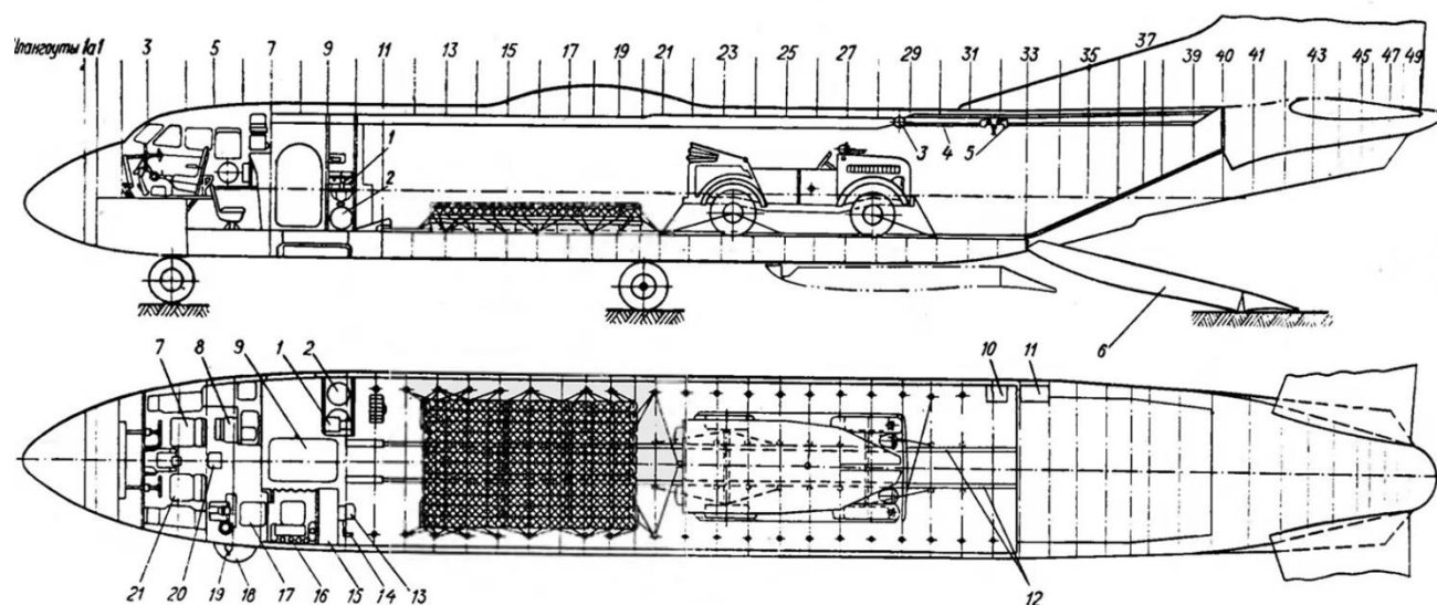
Рис. 2. Компоновочная схема кабины самолета:
