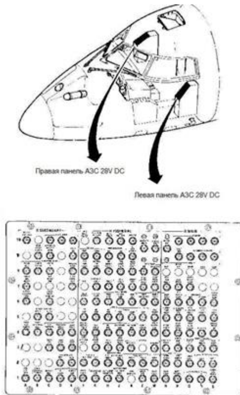
Рис. 69 Расположение панелей А3С 28 В.
